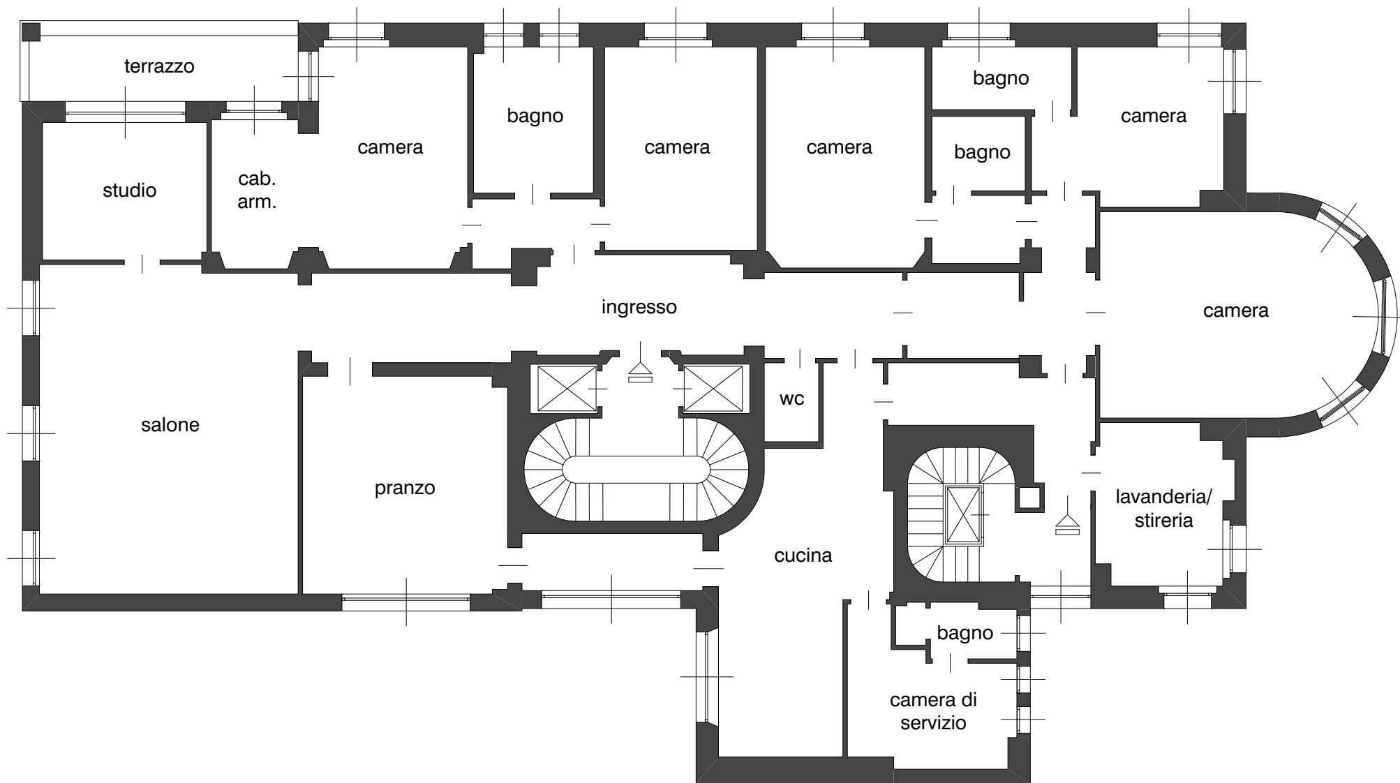
Porta Venezia - secondo piano - stato di fatto
